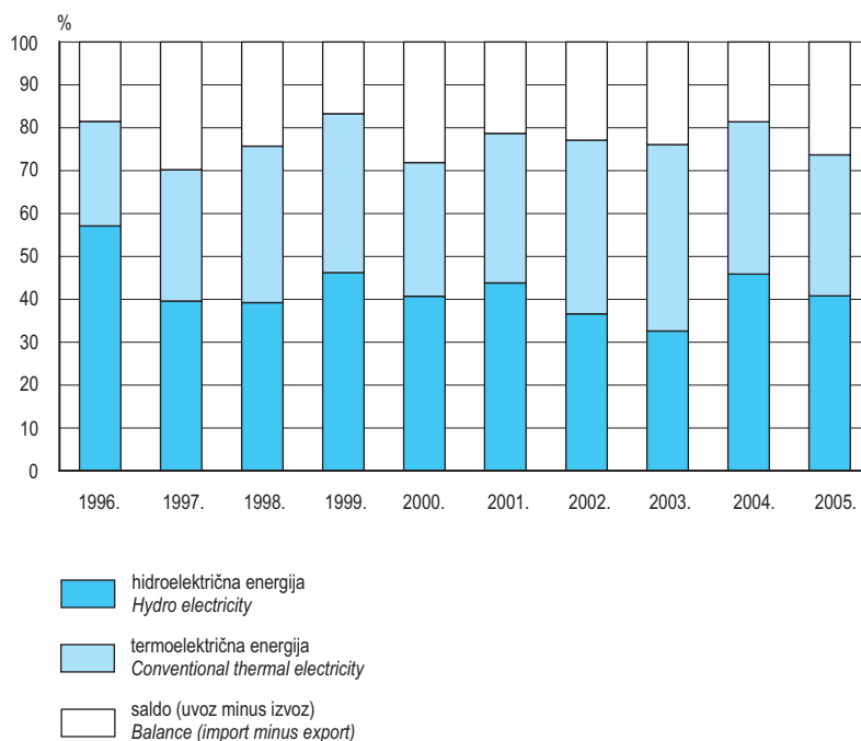
G 18-1. STRUKTURA RASPOLOŽIVE ELEKTRIČNE ENERGIJE OD 1996. DO 2005. STRUCTURE OF AVAILABLE ELECTRICITY 1996 – 2005
